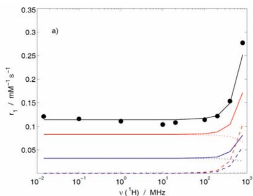
^1\text{H} NMRD profile of [\text{Dy}(\text{CH}_3\text{CN})_9]^{3+} in \text{CH}_3\text{CN} at 298 K.
